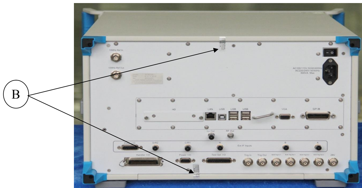
В) Место для пломбировки от несанкционированного доступа Рисунок 2 - Общий вид анализаторов. Вид сзади
